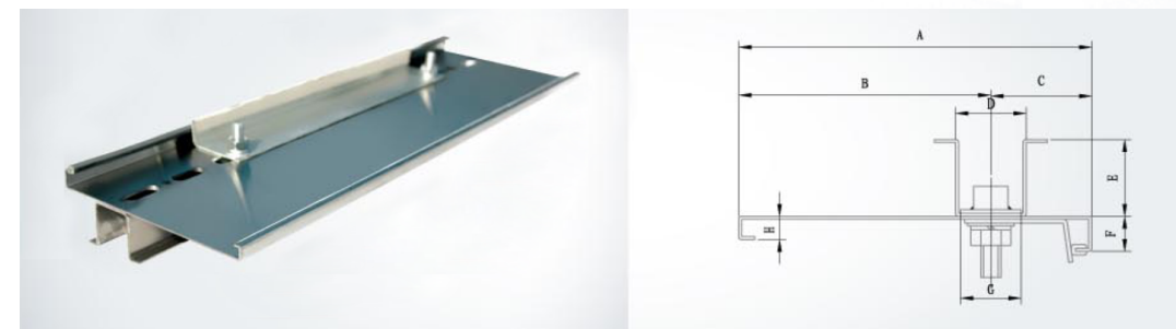
扶手导轨组件 Balustrade guide rail set
